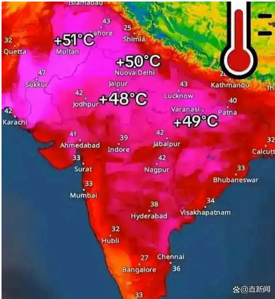
印度近期高温情况。图据直新闻
